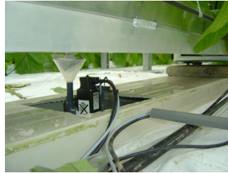
PRIVA GroScale -vaakajärjestelmä ylikastelumittaukseen
